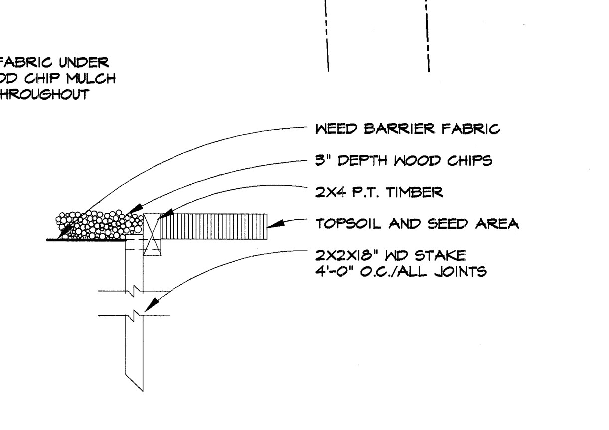
5 2X4 WOOD HEADER DETAIL LI SCALE: NTS
