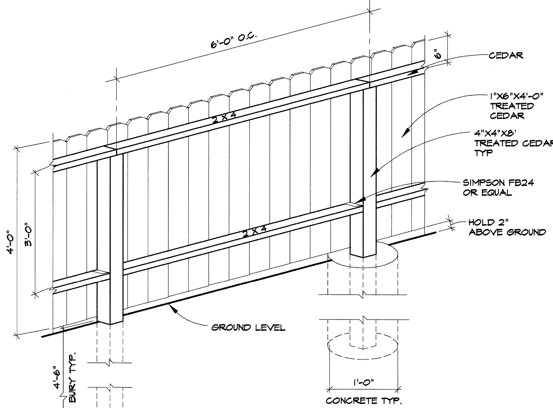
6 FENCE LI SCALE: 3/4" = 1'-0"
